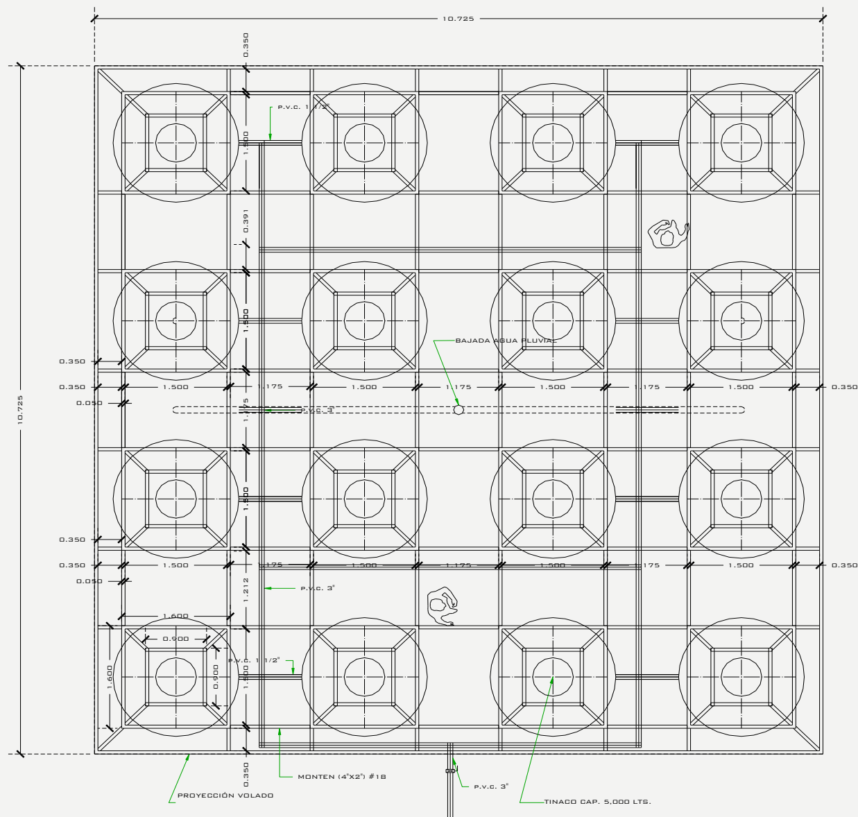
PLANTA ESTRUCTURA
