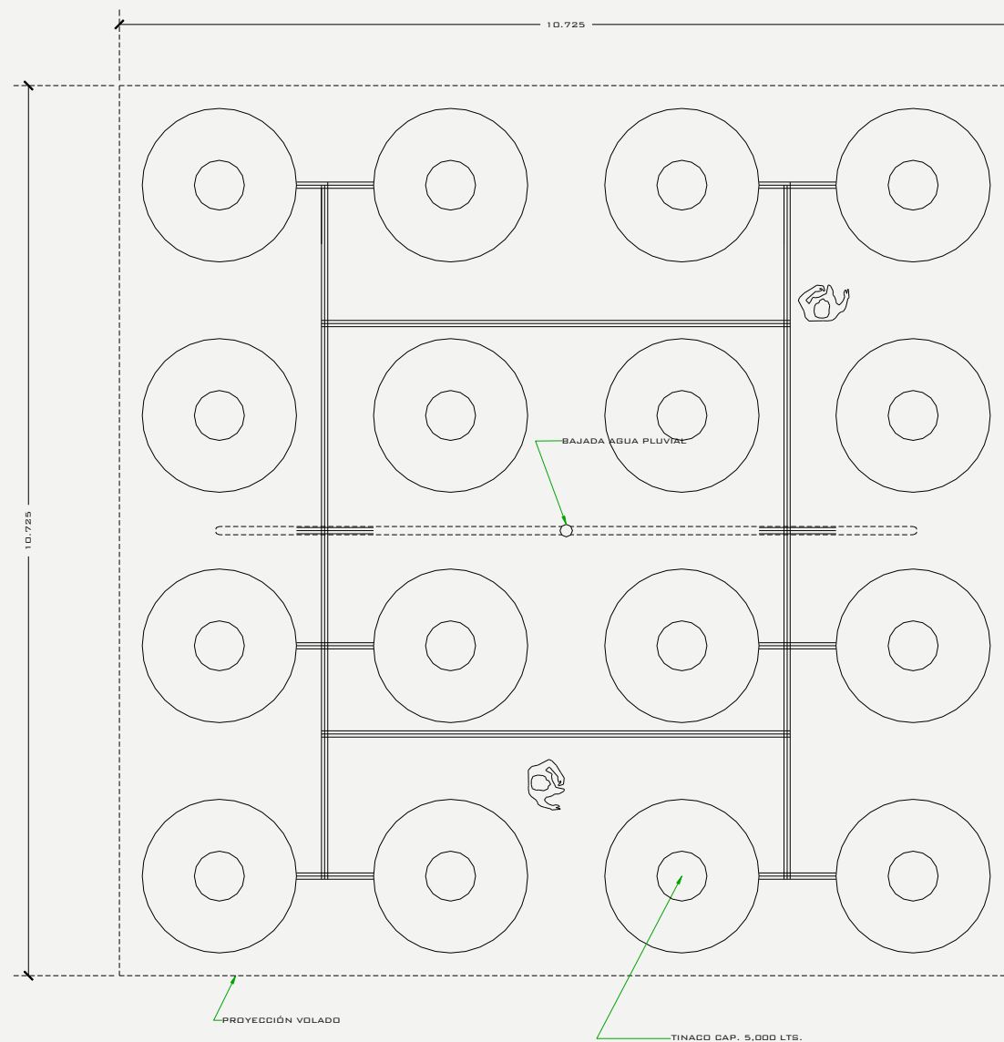
PLANTA ARQUITECTÓNICA
